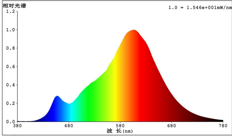
光谱分布
